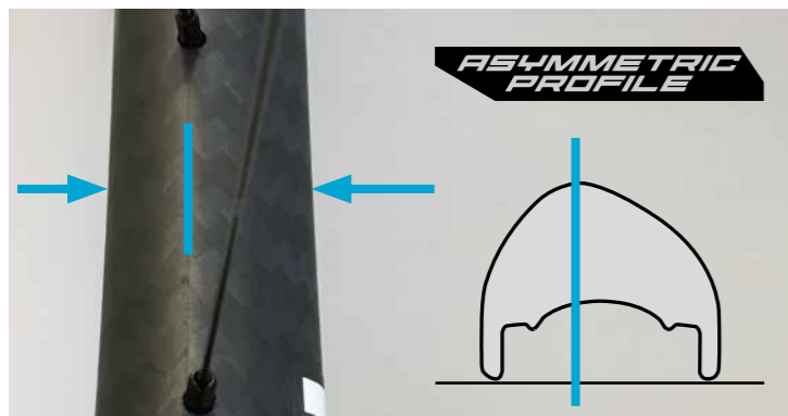
asymmetrisches Felgenprofil / asymmetric rim design
