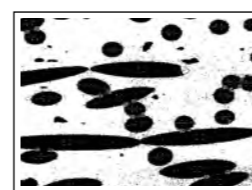
Computerunterstützt verarbeitete optische (vergrößerte) Aufnahme der Oberfläche des Bremsbereiches. / Computer-aided optically processed (enlarged) image of the surface of the brake sector.
