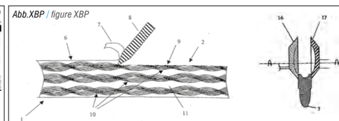
Abb.XBP / figure XBP Abb. XBP zeigt die typische Materialbeschaffenheit des Verbundmaterials nach dem Urformprozess in der Felgenflanke vor und nach der erfindungsgemäßen Bearbeitung. / Fig. XBP shows the typical nature of the composite material after the primary shaping process in the rim edge before and after processing according to the patented labor process.
